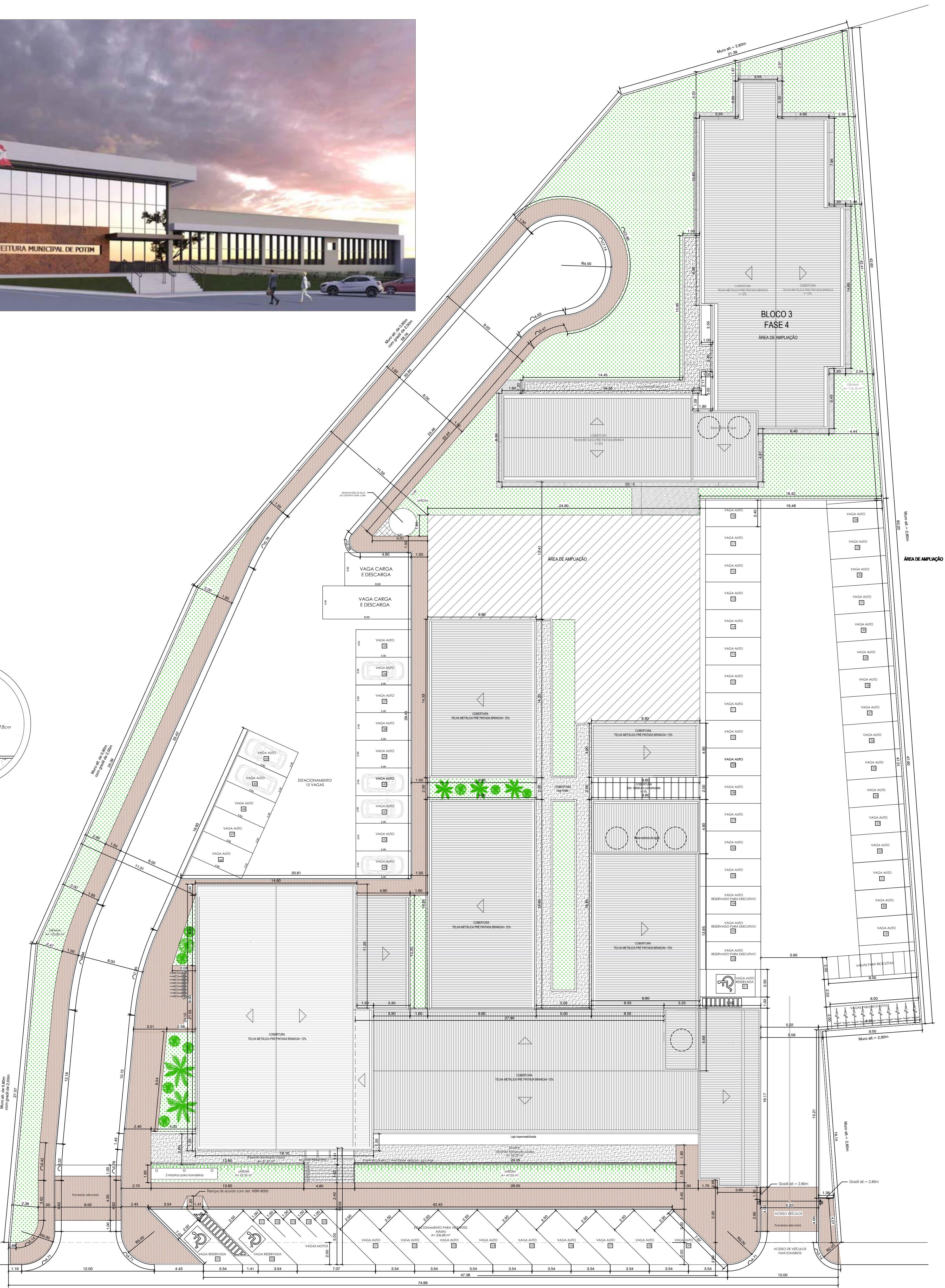
IMPLANTAÇÃO ESC. 1:100
